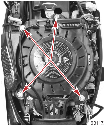
Quatre vis et rondelles fixant le lanceur
