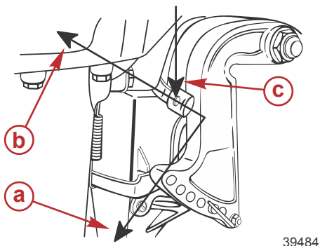
a - Position d'abaissement b - Position de relevage c - Levier de blocage en marche arrière
