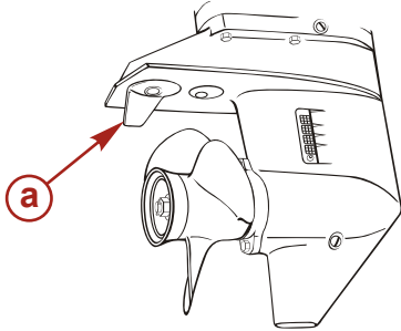
a - Anode/dérive
