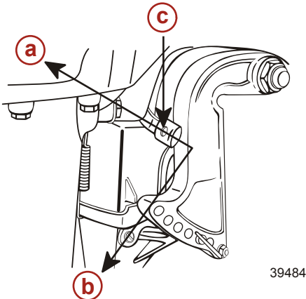
a - Position d'abaissement b - Position de relevage c - Levier de blocage en marche arrière
