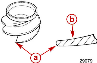
a - Bord d'attaque b - Angle de levage supérieur
