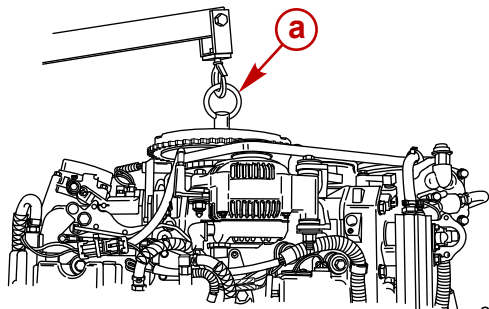
a - Anneau de levage
