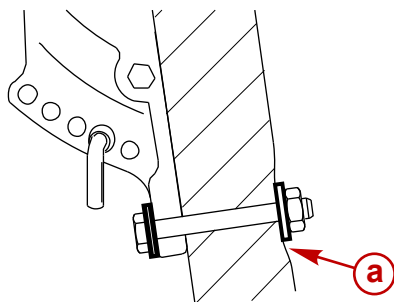
a - Tableau arrière cédant sous le couple du boulon
