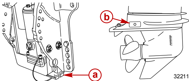
a - Anode sur bras de tableau arrière
