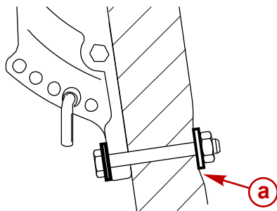
a- Tableau arrière cédant sous le couple de la vis
