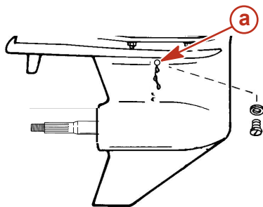
a - Évent
