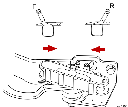
Moteur hors-bord à contre-rotation
