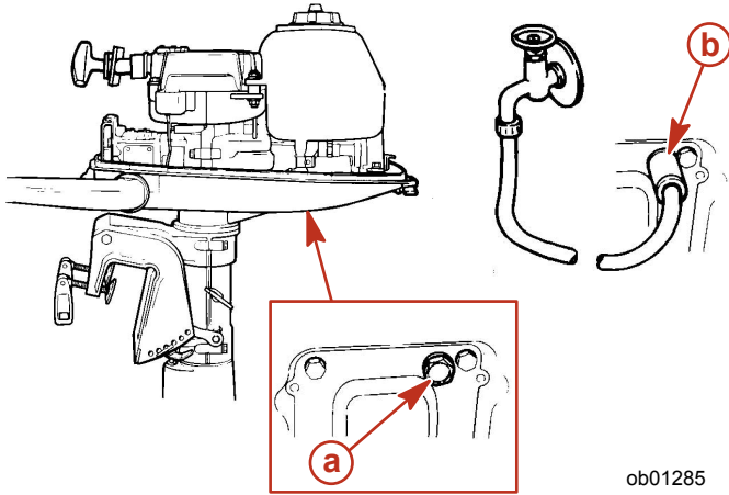
a- Bouchon et joint d'étanchéité
