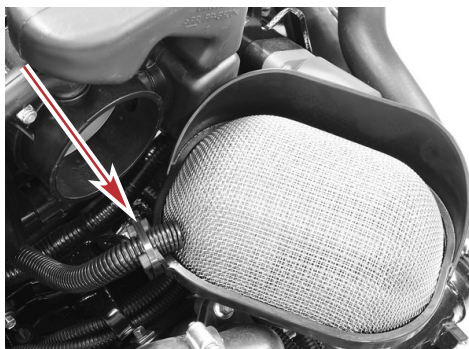
Tuyau d'évent du carter-moteur
