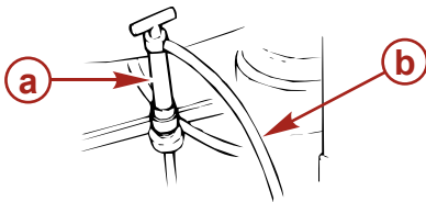
a - Pompe à huile de carter de moteur b - Tuyau de pompe à huile de carter de moteur
