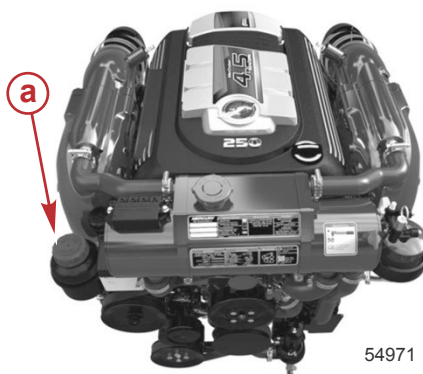
Bouchon de remplissage/jauge.
