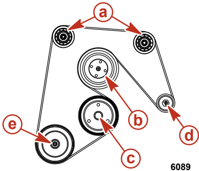
a - Poulie folle b - Poulie de la pompe de circulation c - Poulie du vilebrequin d - Poulie de l'alternateur e - Poulie de la pompe à eau de mer
