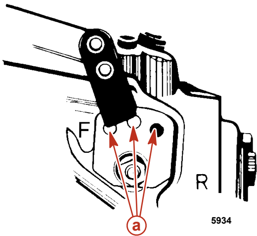
Transmission en ligne a - Bille de verrouillage et orifices
