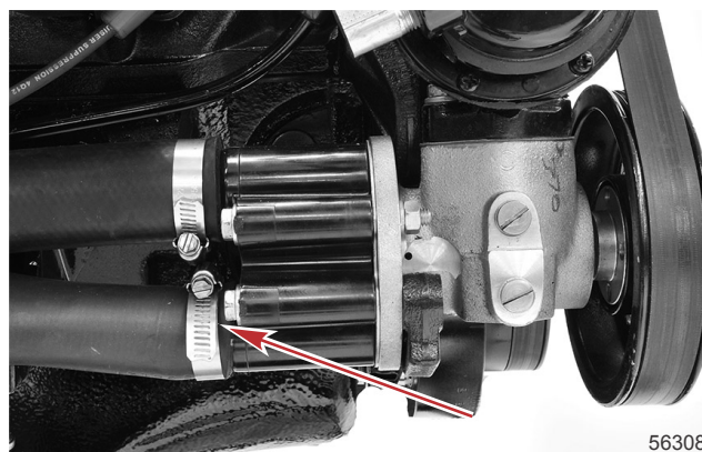
Connexion du tuyau d'arrivée d'eau de mer
