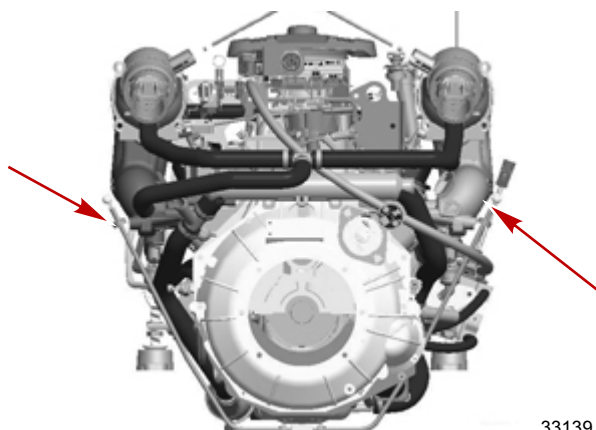
Emplacements possibles de la jauge d'huile – Modèles 5.7, 6.2 MPI ECT, Horizon 5.7, 6.2 ECT
