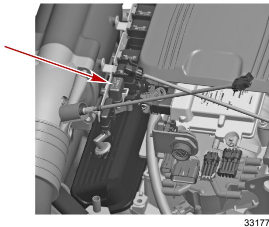
Fusibles de capteurs d'oxygène
