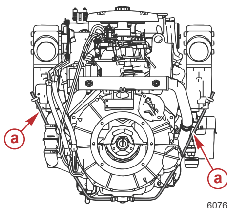
a - Tube de la jauge d'huile
