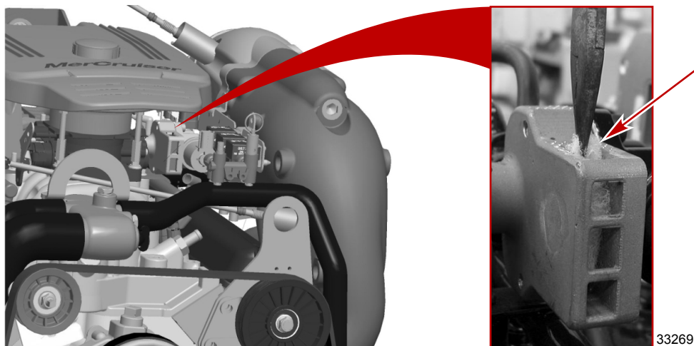
Le silencieux de régulation d'air de ralenti est installé dans l'adaptateur de régulation d'air de ralenti
