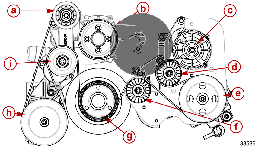
Schéma d'acheminement de la courroie
