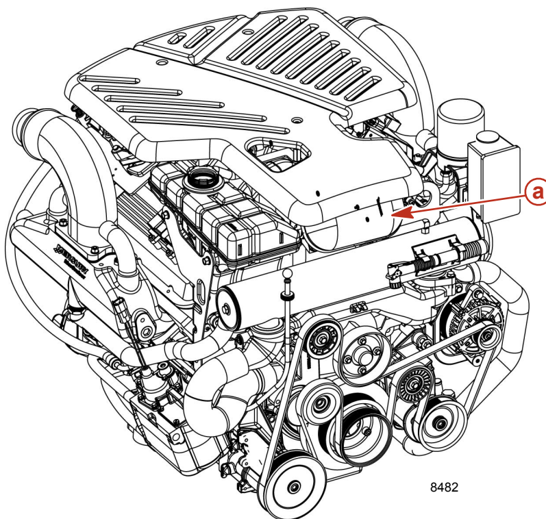
a - Pare-flammes
