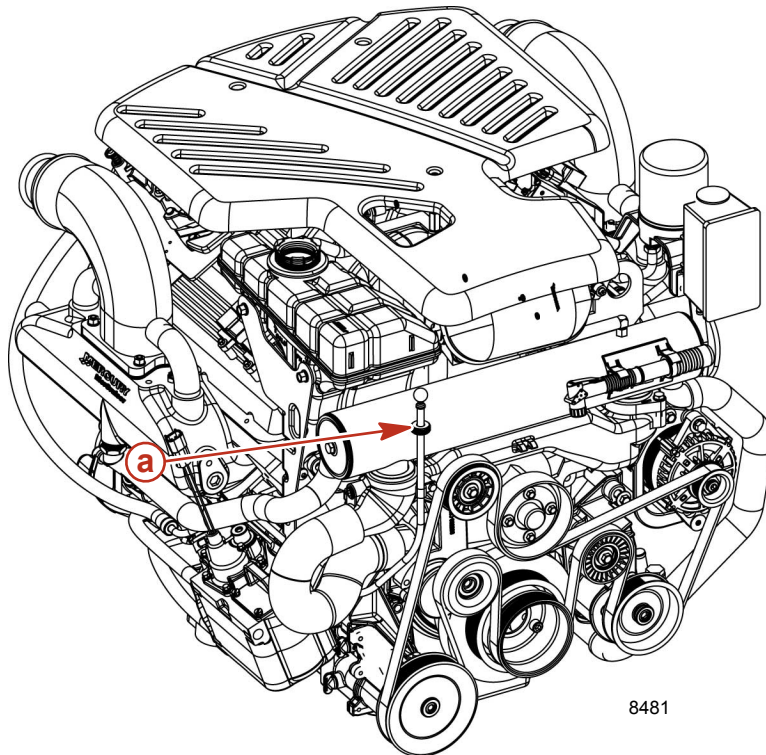
a - Tube de la jauge d'huile
