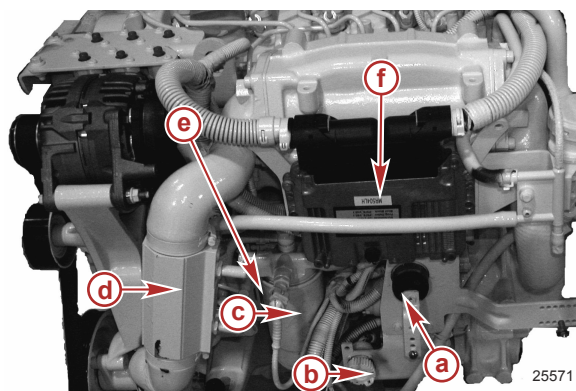
Côté bâbord du moteur
