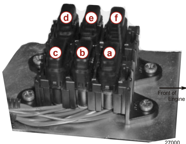
Panneau de fusible de moteur de 2.0 I
