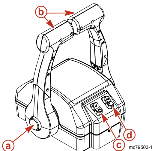
c - Bouton de relevage hydraulique d - Bouton de relevage pour transport sur remorque
