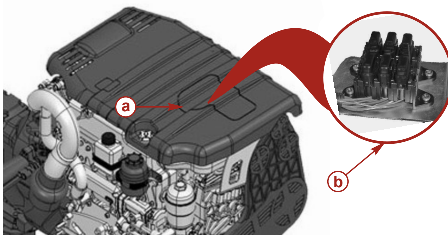
Capot de moteur de 2.0 I avec panneau d'accès
