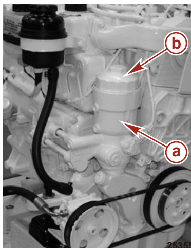
Emplacement du logement du filtre à huile du modèle 2.0L
