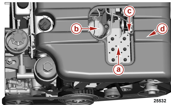
Capot moteur QSD 2.0L avec panneau d'accès retiré
