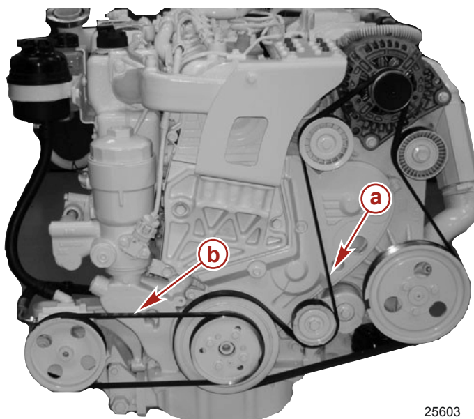
Modèle QSD 2.0 L capot moteur retiré
