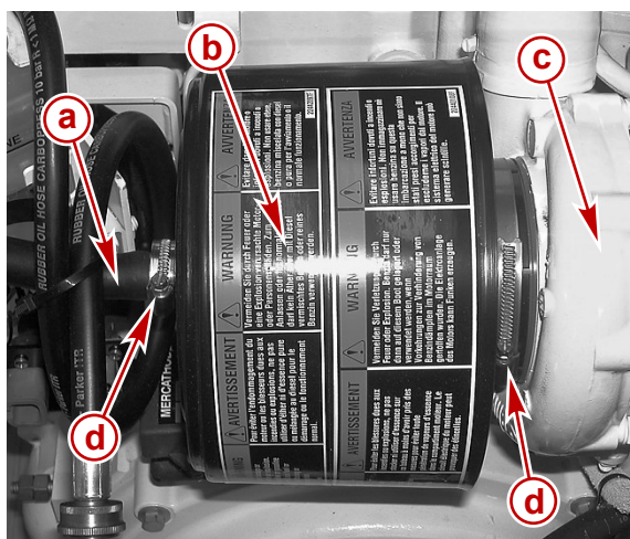
25881 a - Tuyau de l'évent du séparateur d'huile c - Turbocompresseur b - Logement du filtre à air d - Collier de retenue
