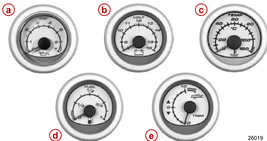
Instruments typiques
