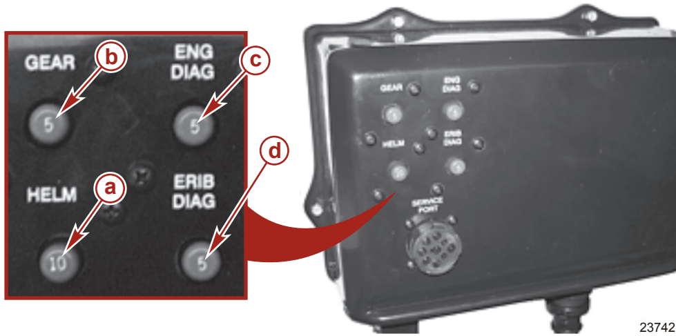
Coupe-circuits du panneau d'intégration du bateau (VIP)
