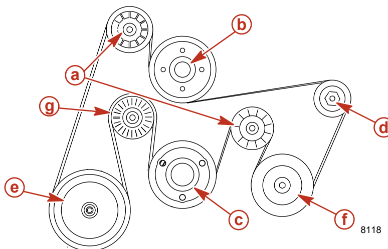
Schéma d'acheminement de la courroie
