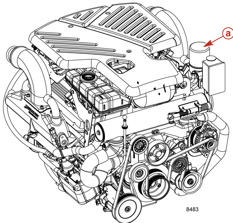
a - Filtre à huile
