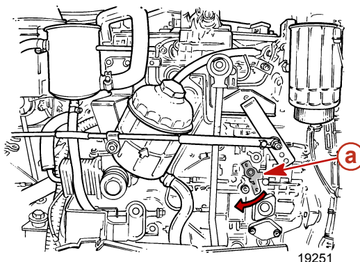
a - Levier d'arrêt du moteur mécanique
