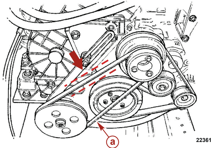
a - Courroie de pompe de direction assistée
