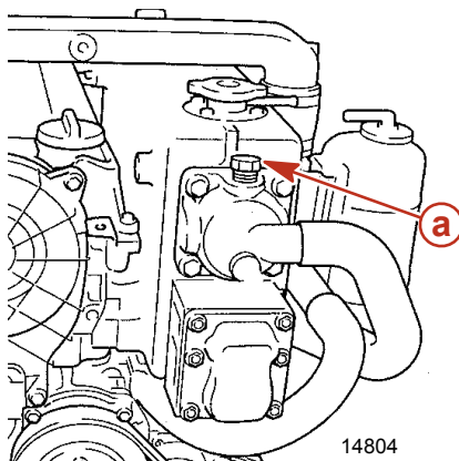
a - Bouchon à anode
