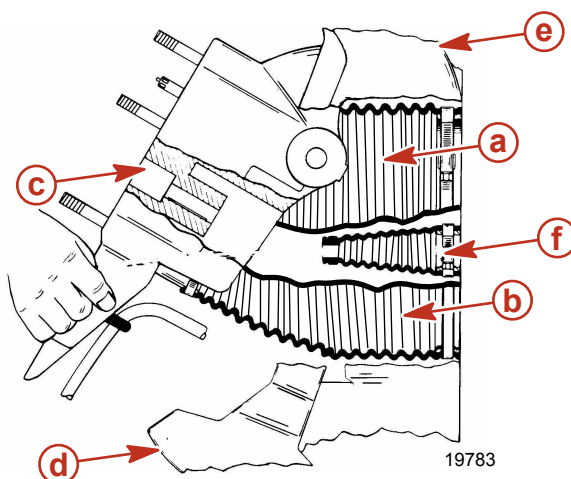
a - Soufflet de joint de cardan d - Anneau de cloche b - Soufflet d'échappement e - Carter de cloche c - Carter de transmission f - Soufflet du câble d'inversion de marche
