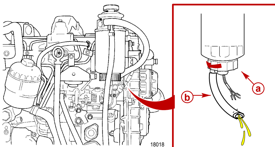
a - Bouchon de vidange
