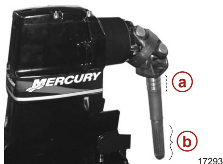
a - Joints toriques (3) de joint de cardan b - Cannelures de l'arbre moteur
