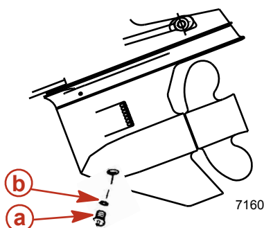
a - Vis de remplissage/vidange d'huile b - Rondelle d'étanchéité
