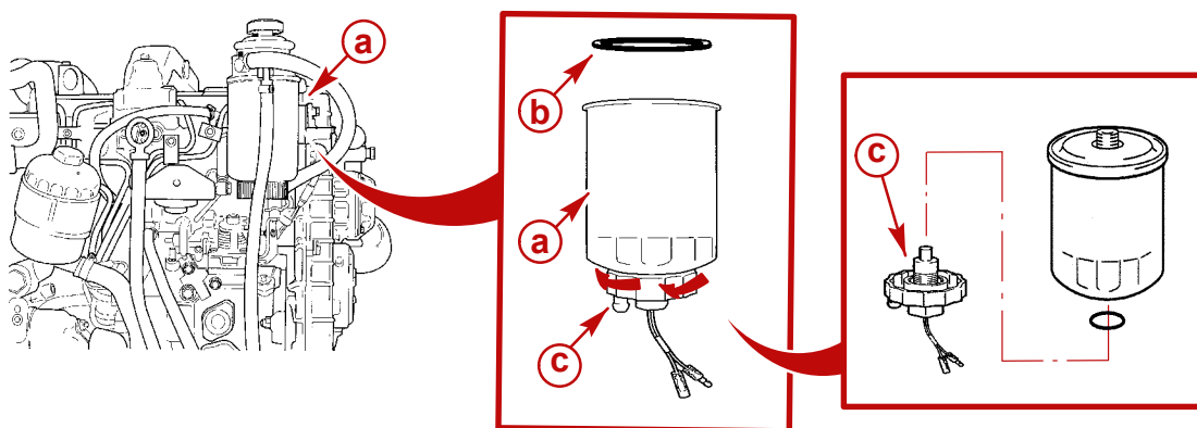
a - Filtre à carburant à séparateur d'eau
