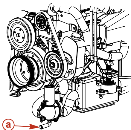
a - Emplacement de l'orifice de vidange bâbord
