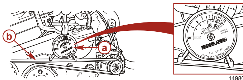
a - Jauge de tension Kent Moore
