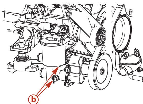
b - Emplacement de l'orifice de vidange tribord
