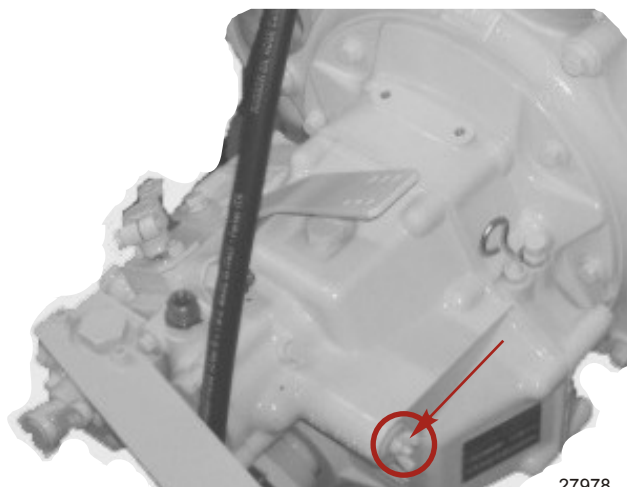
Tuerca de retención del filtro de aceite de la transmisión
