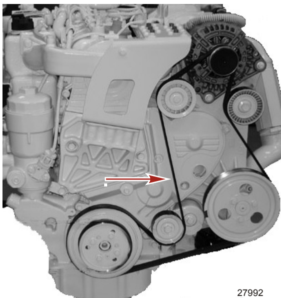
Correa de transmisión serpentina de QSD 2.0
