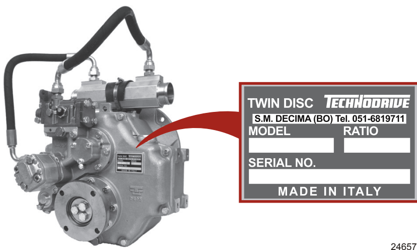
Placa de identificación de Technodrive TM 485-A
