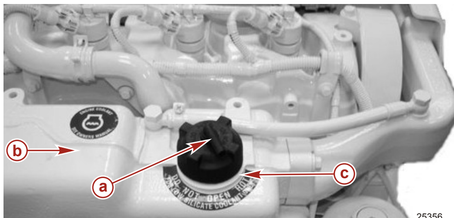
Ubicación de la tapa del refrigerante del motor (con la cubierta del motor extraída)
