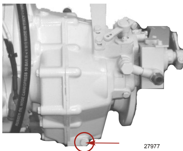
Tapón de drenaje de la transmisión
