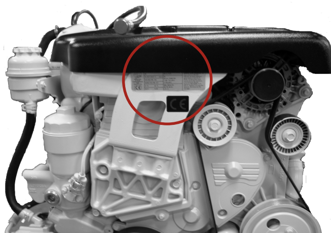
Ubicación de la placa de datos del motor QSD 2.0
