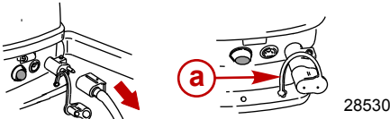
a - Protector cap
