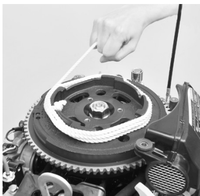
Notstartseil am Schwungrad
