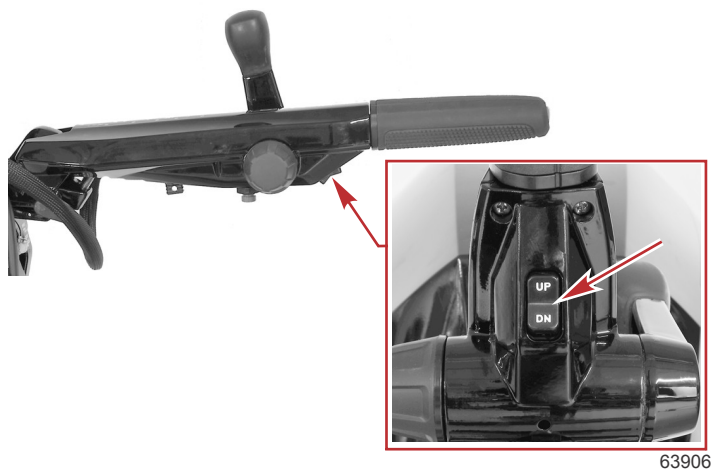
Kippschalter an Modellen mit Ruderpinne
