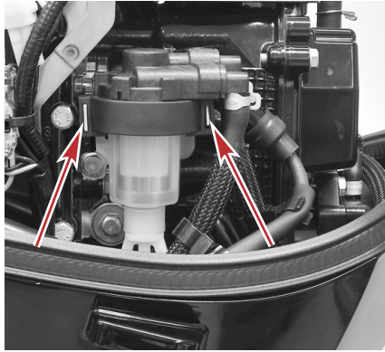
Filter-Montagehalter
