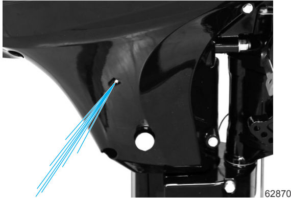
Wasserpumpenkontrolldüse
