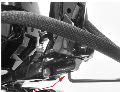
6-mm-Innensechskant-Gelenkschraube
