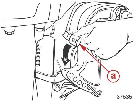
a - Rückfahrsperrhebel
