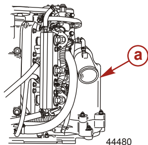
a - Expansionskammer
