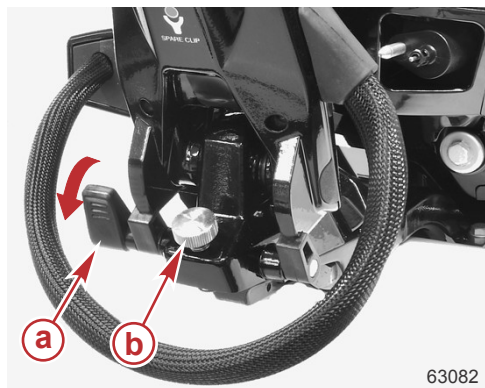
a. Einstellknopf in der niedrigsten Einstellung.
