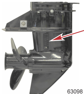
Kühlwassereinlass
