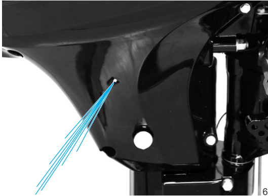
Wasserpumpenkontrolldüse
