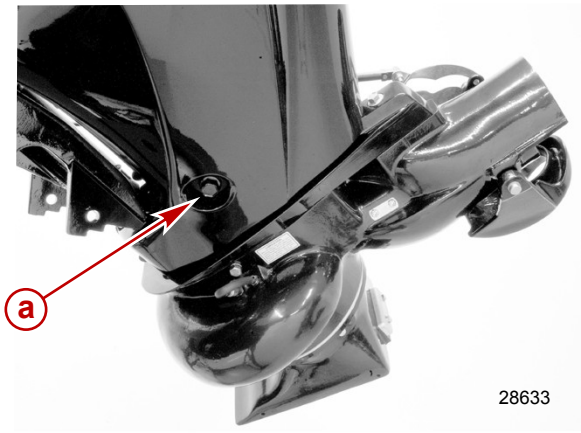
a - Ablassschraube
