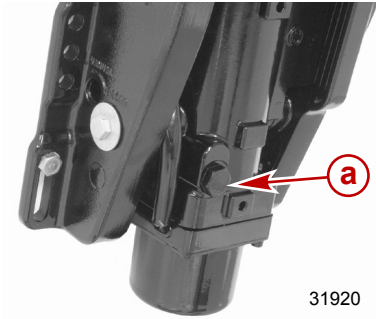
a - Einfülldeckel
