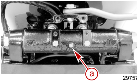
a - Kipprohr-Schmiernippel
