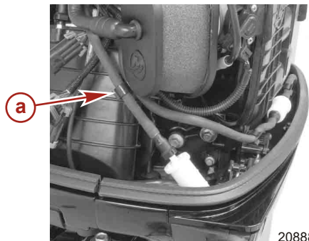
a - Kraftstoffschlauchhalterung
