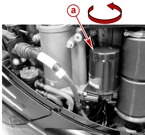
a - Ölfilter
