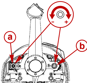
a - Raststellungs-Spannschraube b - Bedienhebel-Spannschraube
