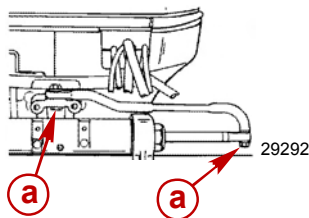
a - Selbstsichernde Muttern
