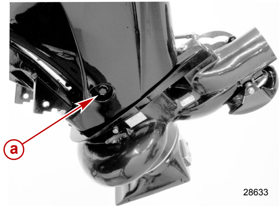
a - Ablassschraube
