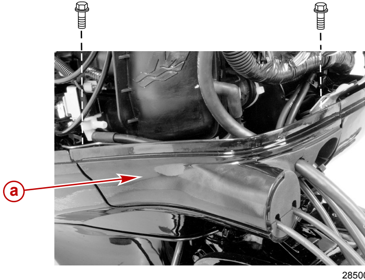
a - Zugangsdeckel
