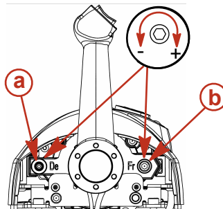
b - Bedienhebel-Spannschraube
