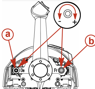
b - Bedienhebel-Spannschraube
