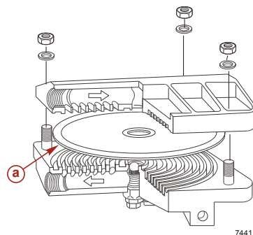
a - Oberg Siebfilter
