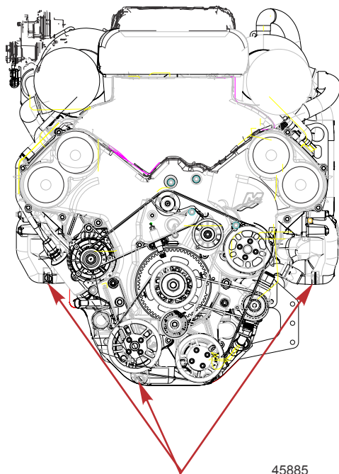
Drei Ablassschrauben für den Seewasserteil
