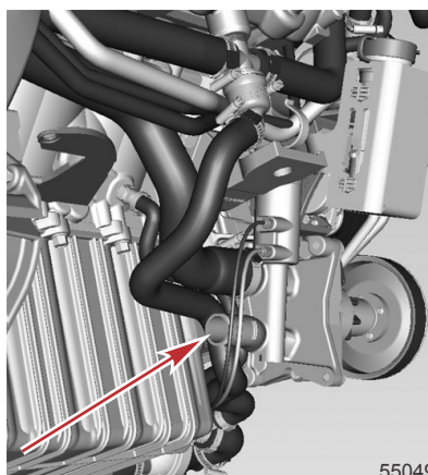
Anschluss des Seewasser-Einlassschlauchs
