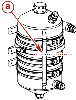
a - Ölbehälter-Schauglas
