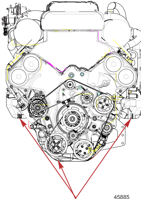
Drei Ablassschrauben für den Seewasserteil
