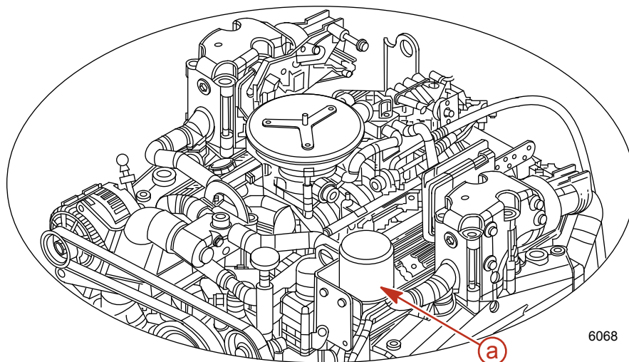
a - Ölfilter
