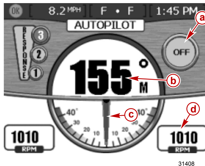
VesselView Standby-Anzeige
