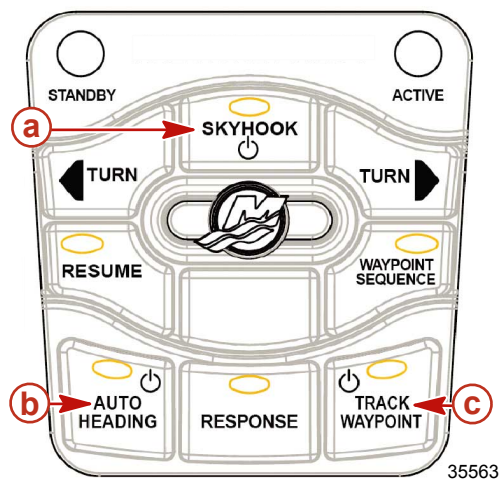
a - „SKYHOOK“-Taste
