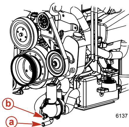
a - Lage des Ablasses – orange oder rot b - Blauer Ablassstopfen
