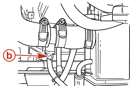
b - Schlauch vom Kraftstoffkühler zum Thermostatgehäuse
