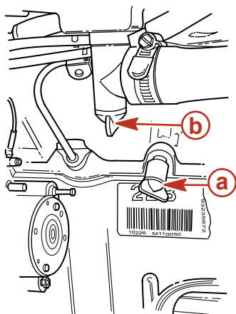
a - Zylinderblock-Ablassstopfen
