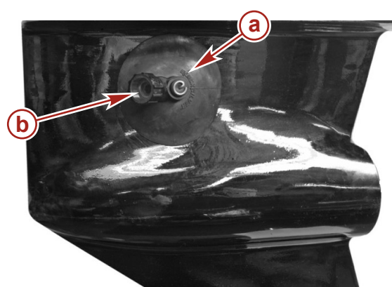
Spülanschlüsse für seitliche Kühlwassereinlässe
