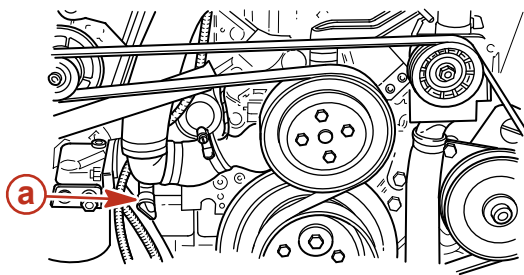
a - Umwälzpumpenschlauch
