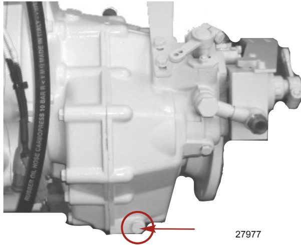
Getriebeöl-Ablassschraube
