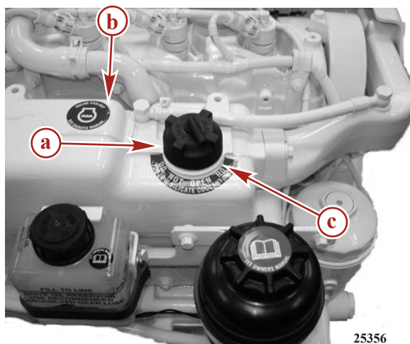
QSD 2.0L (Motorabdeckung entfernt)
