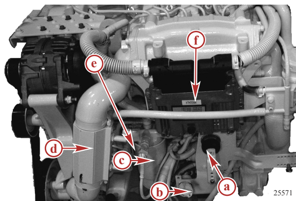
Backbordseite des Motors
