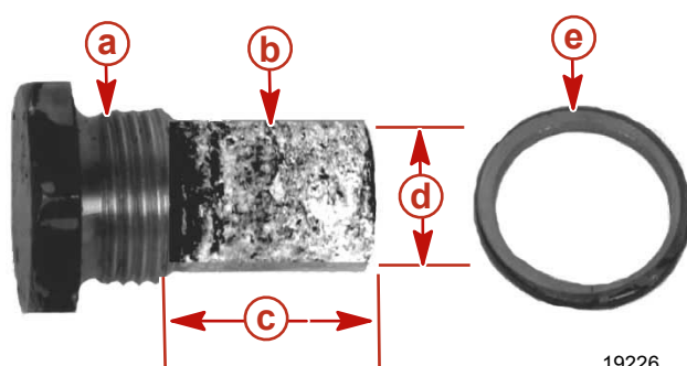
Anode, kpl.
