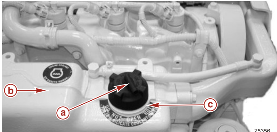
Anordnung des Motorkühlmitteldeckels (Motorabdeckung entfernt)
