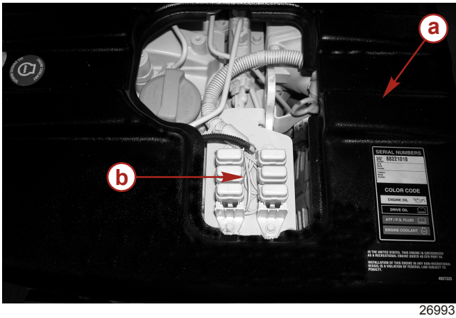
Motorabdeckung mit Zugangsplatte am 2.0 Modell
