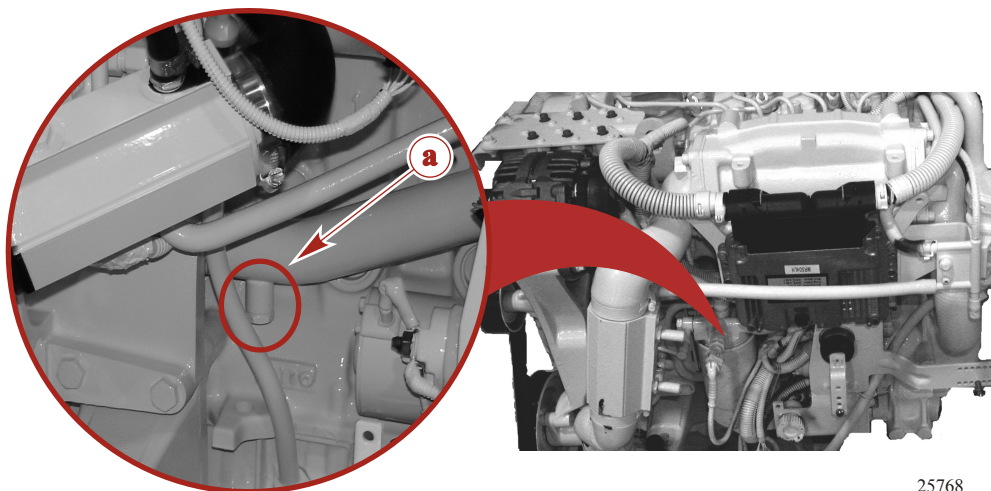
Backbordseite des Blocks mit wasserabscheidendem Kraftstofffilter ausgebaut, um Zugang zu gewährleisten
