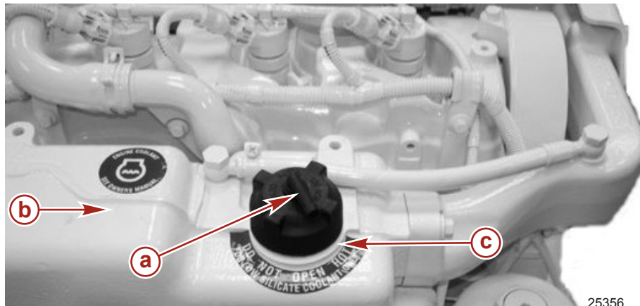
Motorkühlmittel-Einfüllpunkt (Motorabdeckung entfernt)
