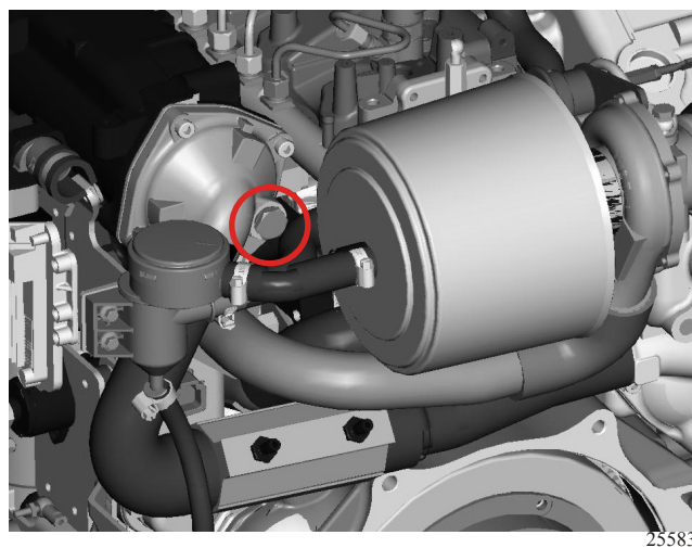
a - Opferanode
