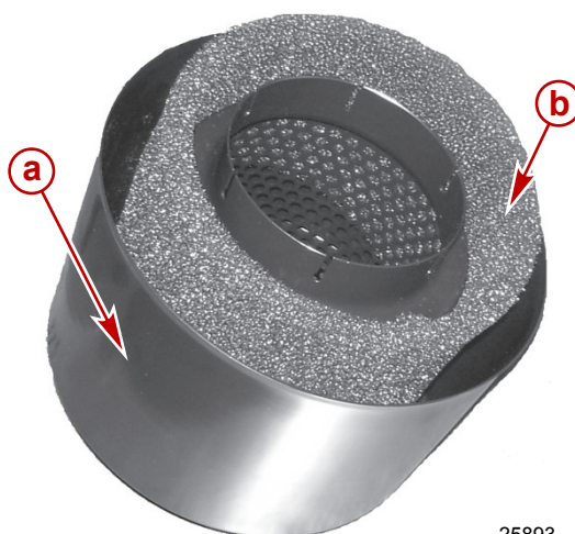
a - Luftfiltergehäuse
