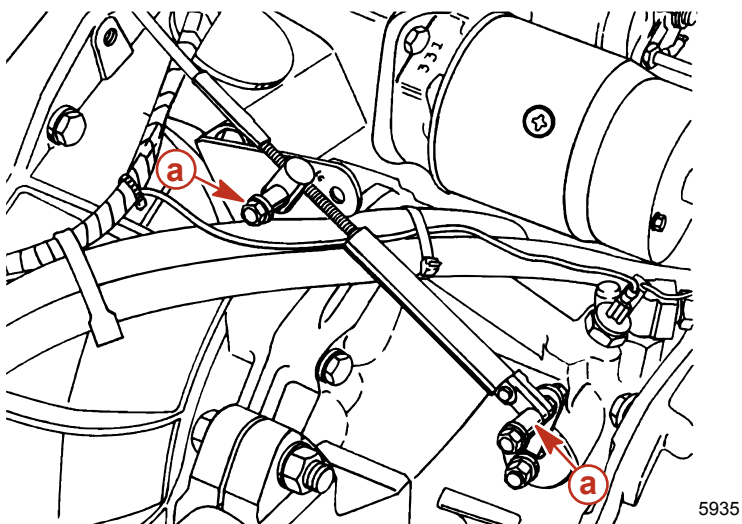
a - Gelenkpunkte
