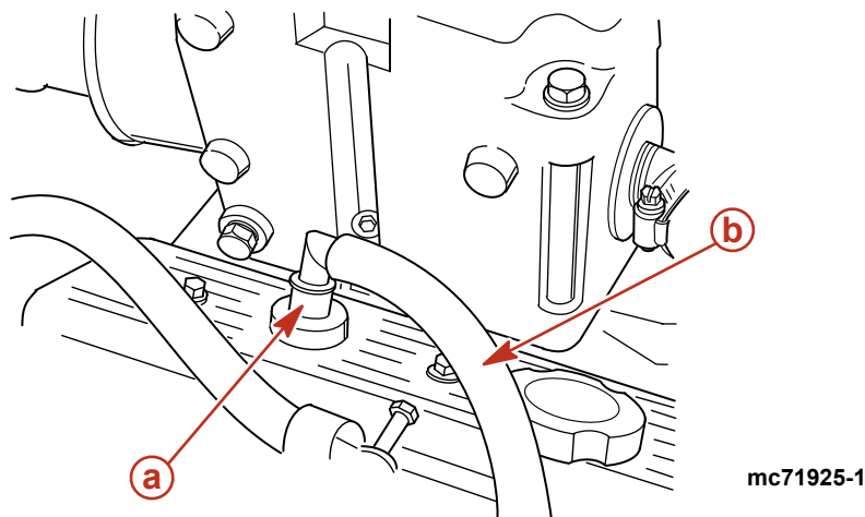
a - PCV-Ventil
