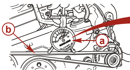
a - Kent Moore® Riemen Spannungsmesser
