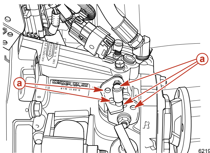
a - Anordnung der Tellerkugel
