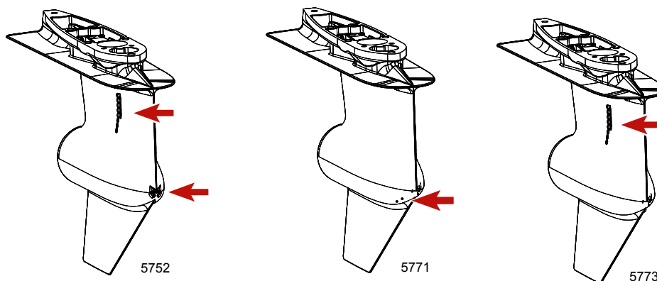
Doppelter Wassereinlass
