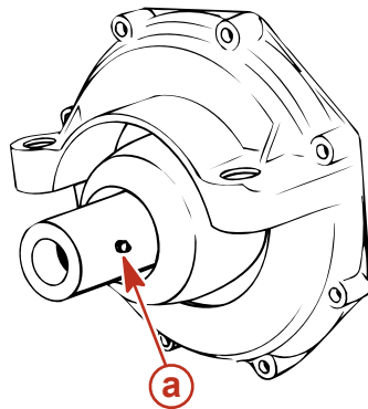
Alpha Antriebskupplung
