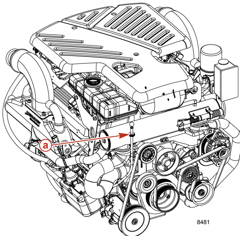
a - Peilstab-Führungsrohr
